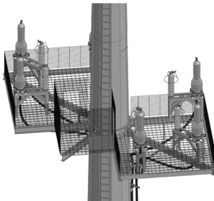
Эксплуатационные площадки на многогранной опоре со шлюзом для подъёма с лестницы на площадку
