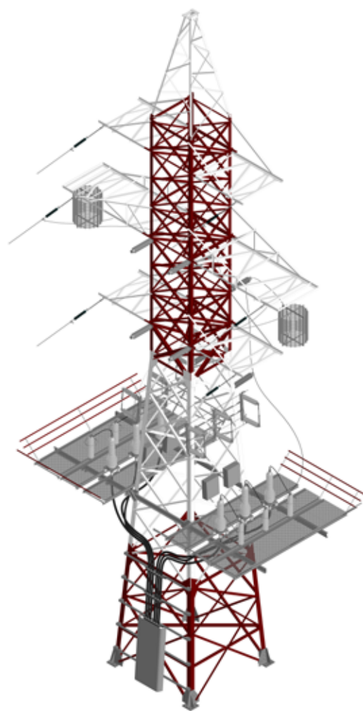
Эксплуатационные площадки на решётчатой опоре
