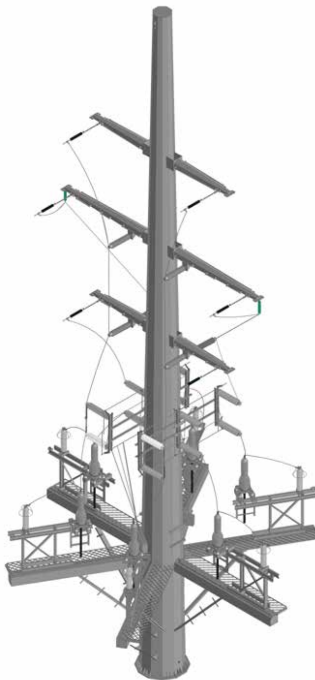
Переходной пункт сверхкомпактной конструкции
