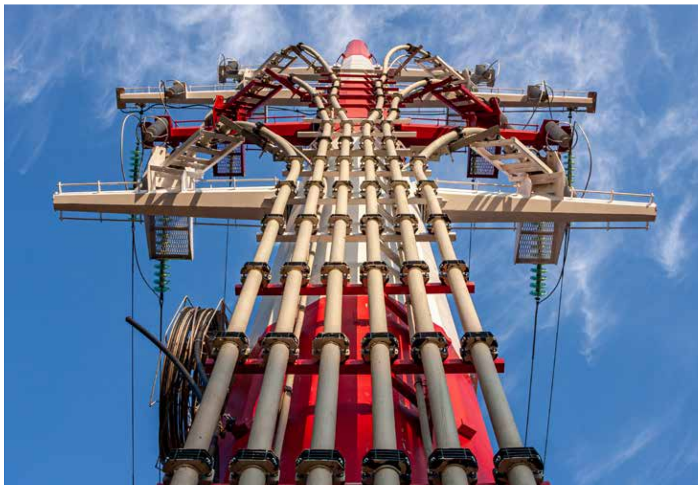
Кабельная лестница и элементы крепления кабеля
